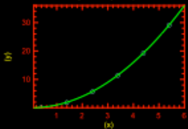
PLplot Example 1 - y=x^2
